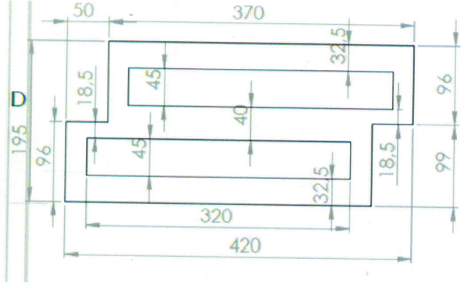
Şekil-1: MEGABLOCK THERMAL/195 mm Görünümü ve Ölçüleri
