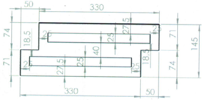
Şekil-1: MEGABLOCK THERMAL/145 mm Görünümü ve Ölçüleri
