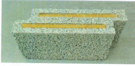
Şekil-1: MEGABLOCK THERMAL/145 mm Görünümü ve Ölçüleri
